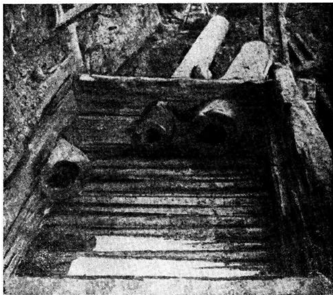
Рис. 3. Водопровод в Новгороде, обнаруженный при раскопках А. В. Арциховским.
